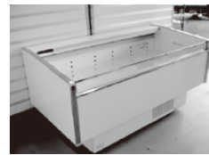
9. 冷蔵オープンケース W1790×D900×H890 240L 電気使用容量:三相200V 1.5KW ¥47,000(税別)
