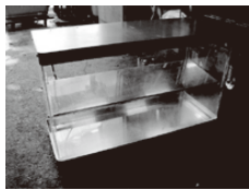
11. ホットケース W750×D300×H550 電気使用容量:約200W ¥32,000(税別)
